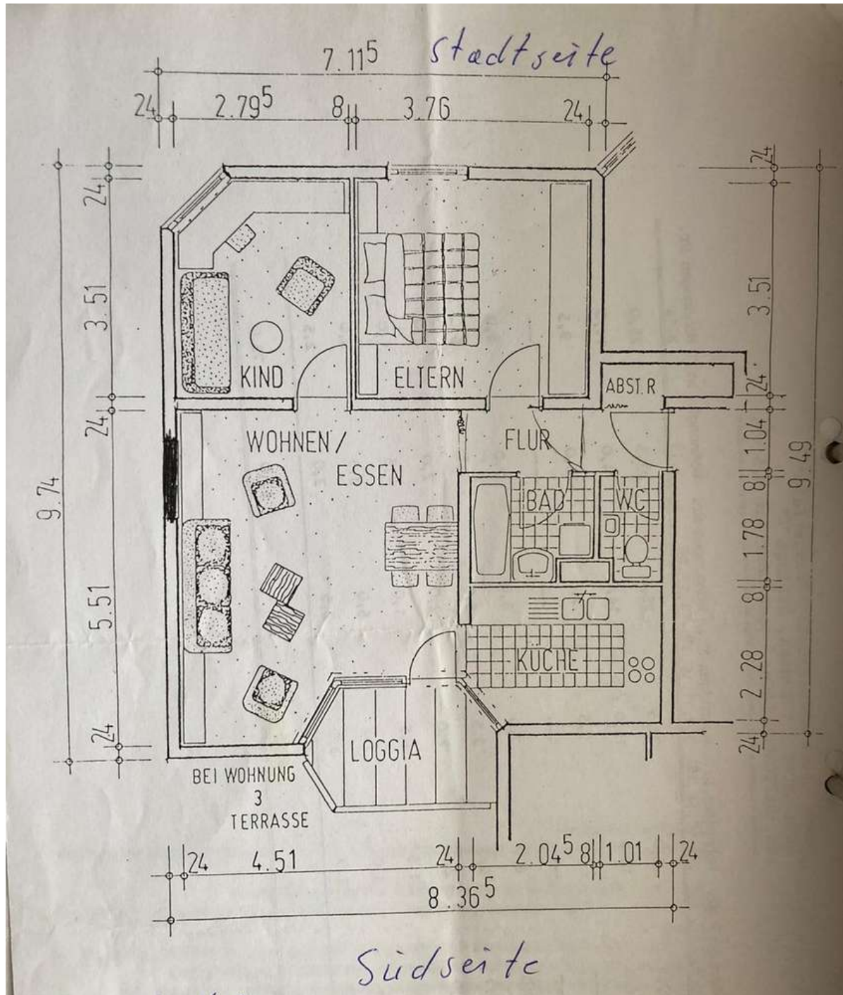
Grundriss
